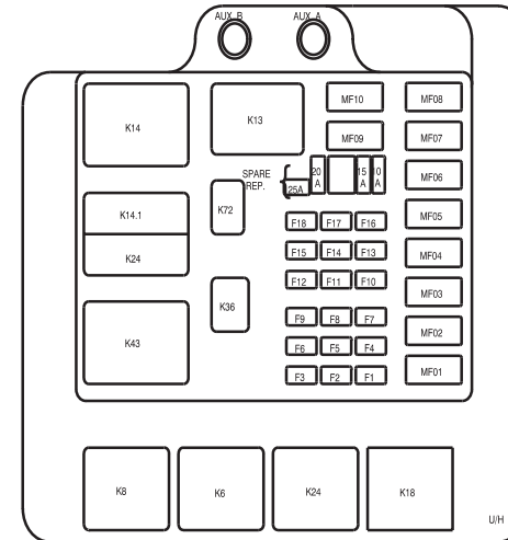
MOTOR 2.4L GASOLINA
