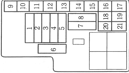
Caixa de Fusível Localizada no Compartimento do Motor
