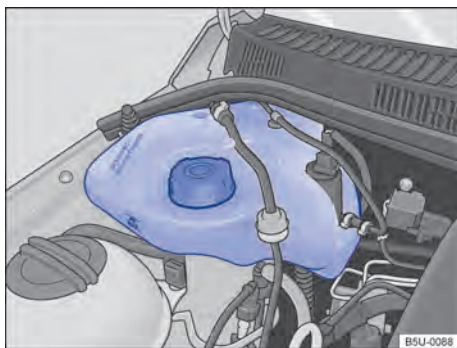
Fig. 132 No compartimento do motor: reservatório de gasolina para o sistema de partida a frio.
