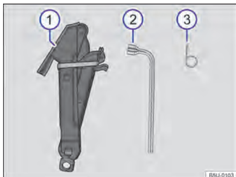
Fig. 104 Componentes das ferramentas de bordo.
