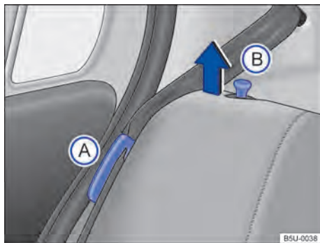
Fig. 56 Banco traseiro: posicionador do cinto de segurança (A) e pino de destravamento do encosto (B).
