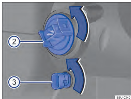
Fig. 108 No compartimento do motor: vista traseira do farol dianteiro (2) indicadores de direção e (3) luz de posição.
