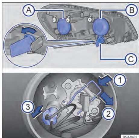
Fig. 110 Acesso à lâmpada incandescente do farol baixo.
