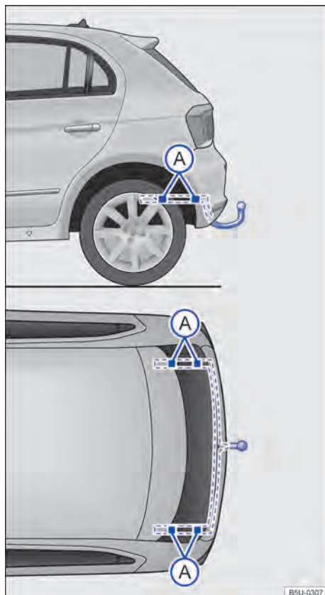
Fig. 100 Pontos de fixação para instalar um dispositivo de reboque posteriormente.
