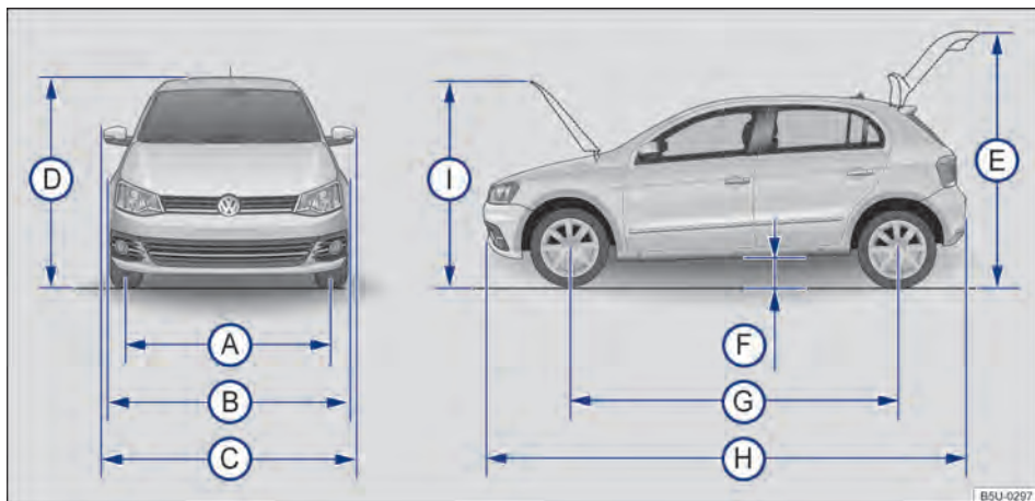
Fig. 153 Dimensões.
