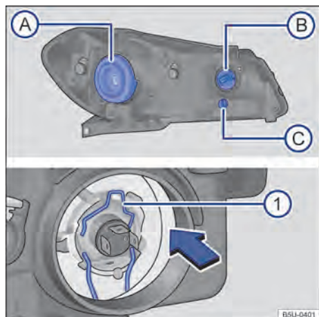
Fig. 107 No compartimento do motor: vista traseira do farol dianteiro com cobertura de borracha (lado esquerdo da ilustração) - (A) farol baixo / alto, (B) indicadores de direção e (C) luz de posição. Vista traseira do farol dianteiro sem a cobertura de borracha (lado direito da ilustração): (1) mola de travamento da lâmpada incandescente do farol baixo / alto.
