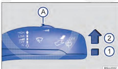
Fig. 73 Alavanca dos limpadores dos vidros: regular a sensibilidade do sensor de chuva A .
