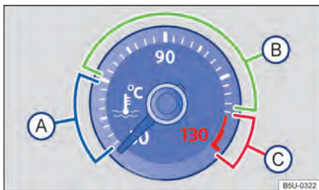
Fig. 38 Indicador de temperatura do líquido de arrefecimento do motor no instrumento combinado (variante 2): (A) área fria; (B) área normal; (C) área de alerta.
