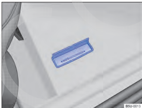
Fig. 176 Em frente ao banco do passageiro dianteiro: número de identificação do veículo (número do chassi) no assoalho, em frente ao banco do passageiro dianteiro.
