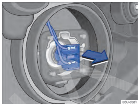
Fig. 134 Acesso à lâmpada incandescente do farol baixo.
