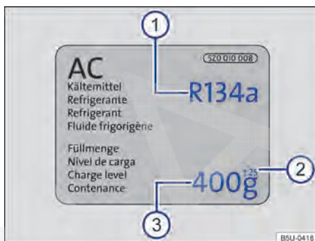
Fig. 178 Informações do ar-condicionado.
