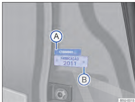
Fig. 177 Na coluna da porta dianteira direita: etiqueta com o número de identificação do veículo parcial (A) e etiqueta de identificação do ano de fabricação (B).
