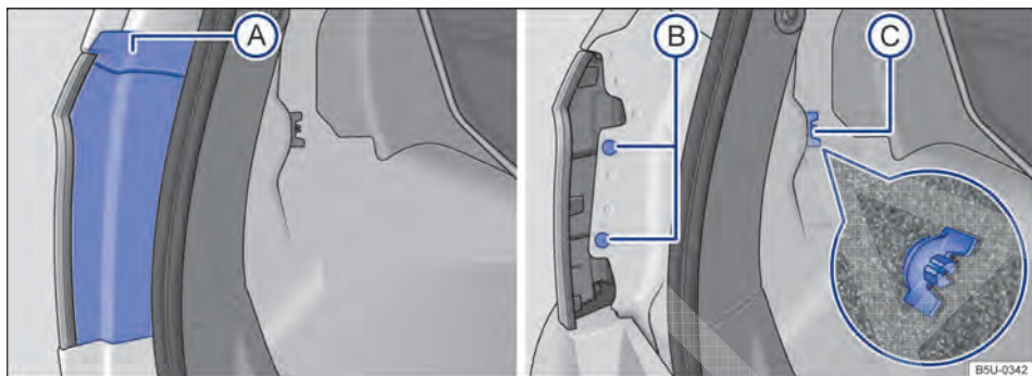
Fig. 136 No compartimento de bagagem: (A) desinstalar cobertura, (B) retirar os dois parafusos de fixação e (C) retirar o parafuso borboleta (lupa).
