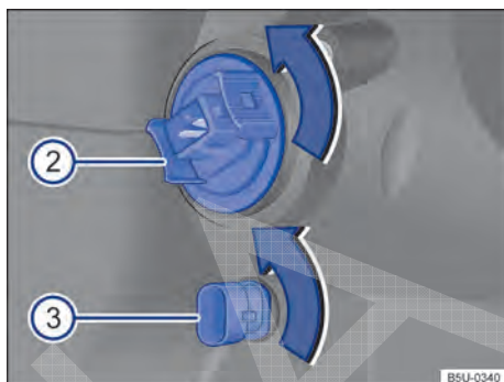
Fig. 132 No compartimento do motor: vista traseira do farol dianteiro 2 indicadores de direção e 3 luz de posição.
