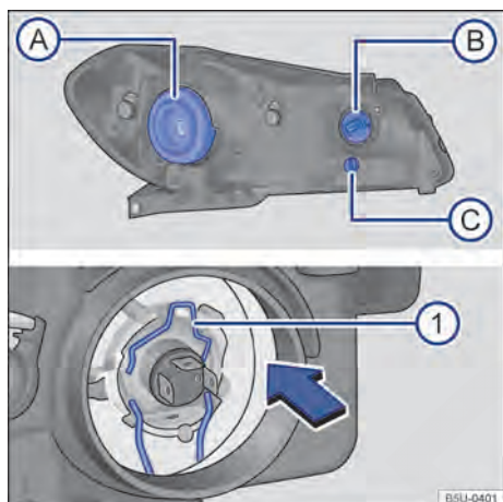
Fig. 131 No compartimento do motor: vista traseira do farol dianteiro com cobertura de borracha (lado esquerdo da ilustração) - A farol baixo / alto, B indicadores de direção e C luz de posição. Vista traseira do farol dianteiro sem a cobertura de borracha (lado direito da ilustração): 1 mola de travamento da lâmpada incandescente do farol baixo / alto.
