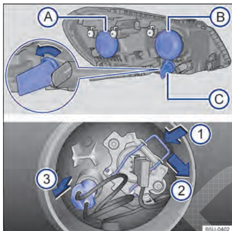
Fig. 134 Acesso à lâmpada incandescente do farol baixo.
