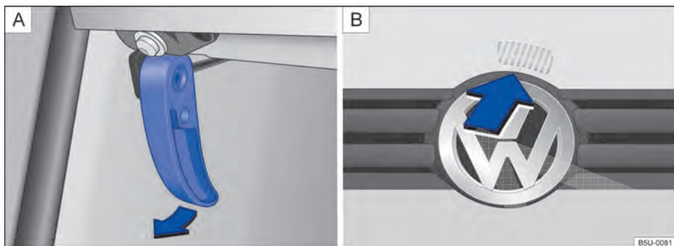
Fig. 148 A ) Alavanca de destravamento da tampa do compartimento do motor na área para os pés do lado do condutor. B ) Alavanca de destravamento na parte interna da tampa do compartimento do motor.
