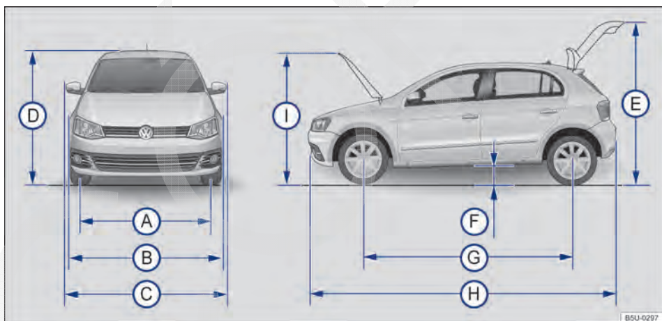
Fig. 179 Dimensões.
