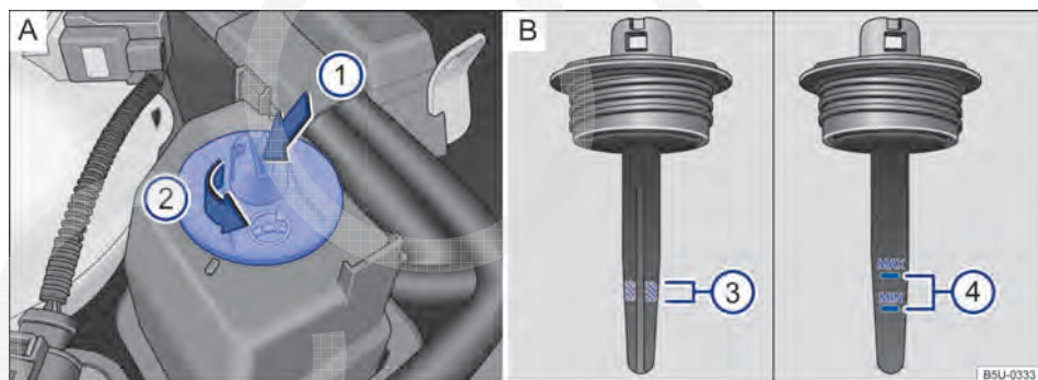
Fig. 99 No compartimento do motor (variante 1): A Reservatório do fluido da direção hidráulica. B Marcações para controle do nível do fluido da direção hidráulica. ▶
