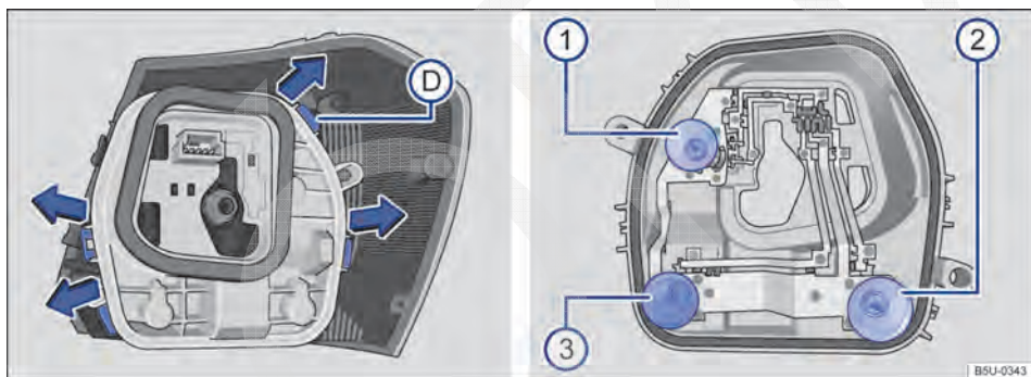
Fig. 137 Lanterna traseira: (D) desinstalar o suporte das lâmpadas e (1), (2) e (3) desinstalar as lâmpadas.
