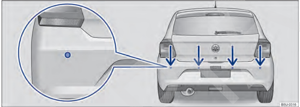
Fig. 109 Sensores de ultrassom do controle de distância de estacionamento no para-choque traseiro.
